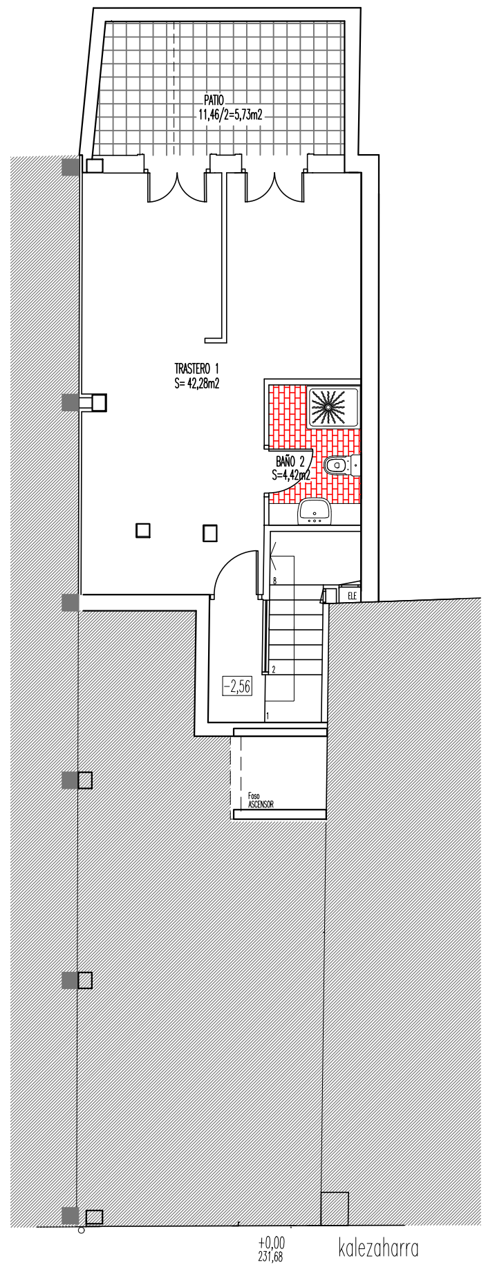
PLANTA SOTANO
